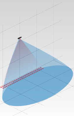
Area detection radar 4 m x 2 m @ 2.2 m infrared 2,2 m x 0,5 m @ 2,2 m
